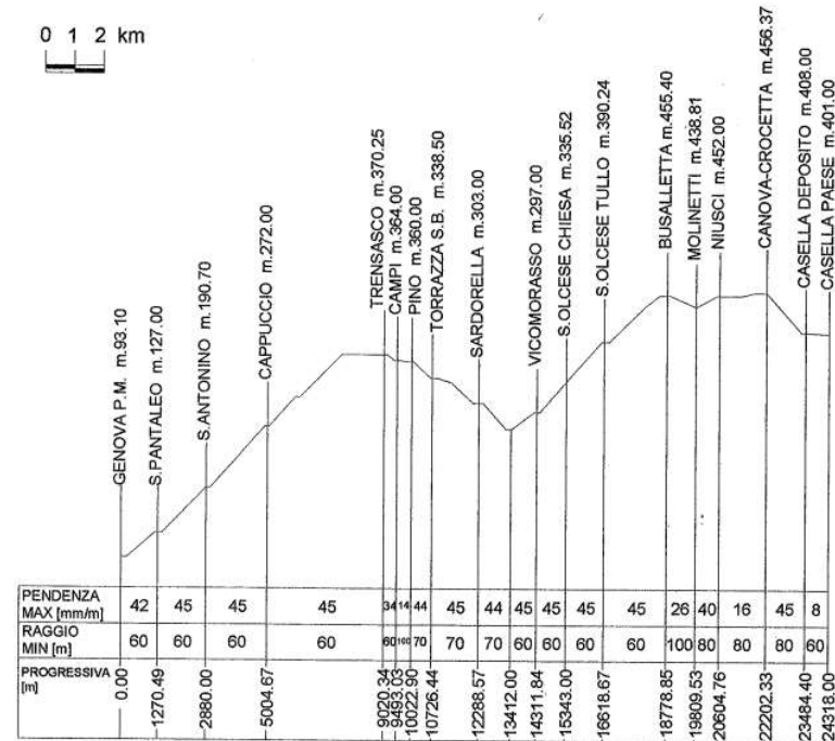
Profilo longitudinale
